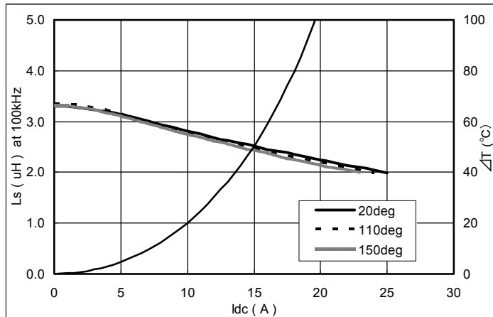
CDMC10D50T150NP-3R3M
