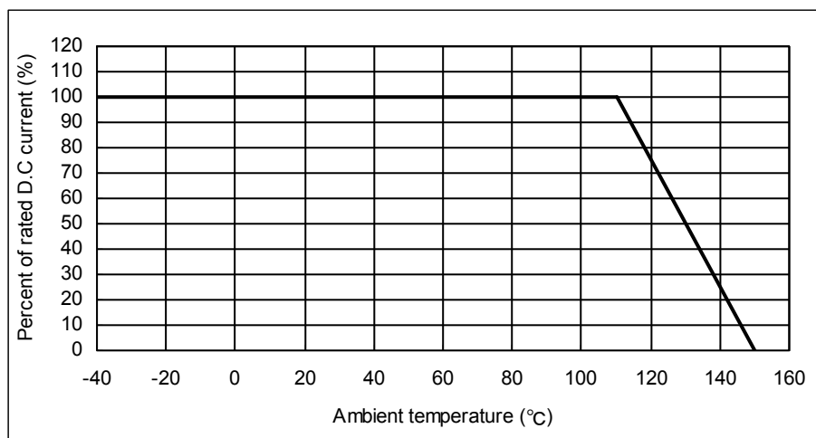
ディレイティング曲線
