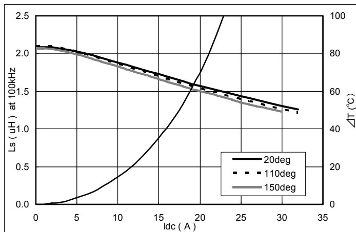
CDMC10D50T150NP-3R3M
